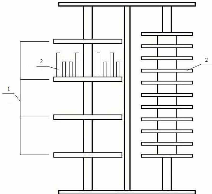
1 – держатели; 2 - инструмент
